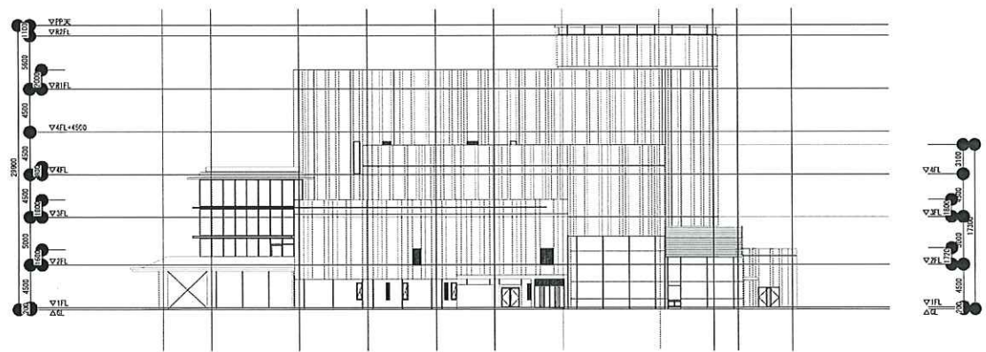
北面 立面図
